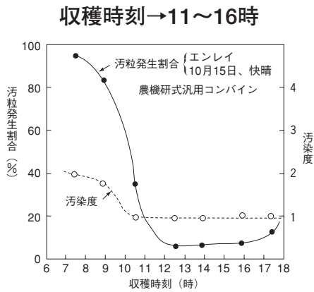
図1. コンバイン収穫における収穫時刻と汚粒発生割合
