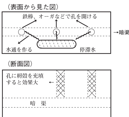
図1. 既設暗きよ活用(籾殻マンホール)
